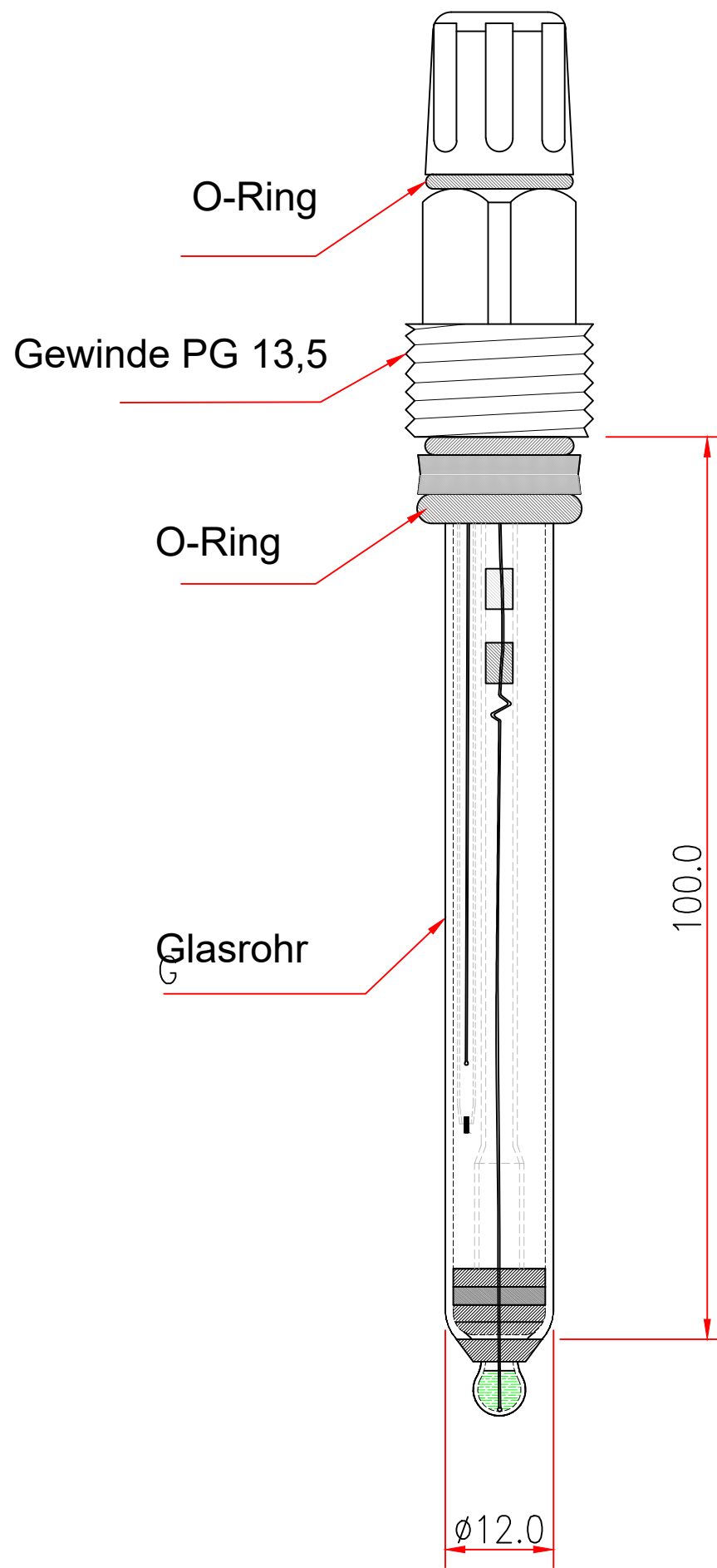
pH Elektrode HBSIGK2-100
